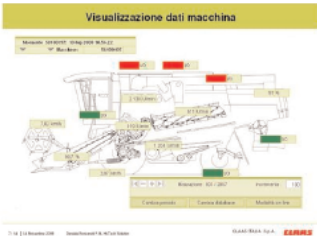
Fig. 19 - Schermata di controllo meccanico di una mietitrebbia del sistema CLAAS Telematics
