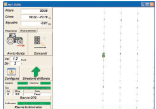
Fig. 12 - Schermata del monitor di controllo della trapiantatrice – Navigazione lungo i filari. (Fonte: Leica Geo) Fig. 12 - Screen of the vine planting machine monitor control - Navigation along the rows.
