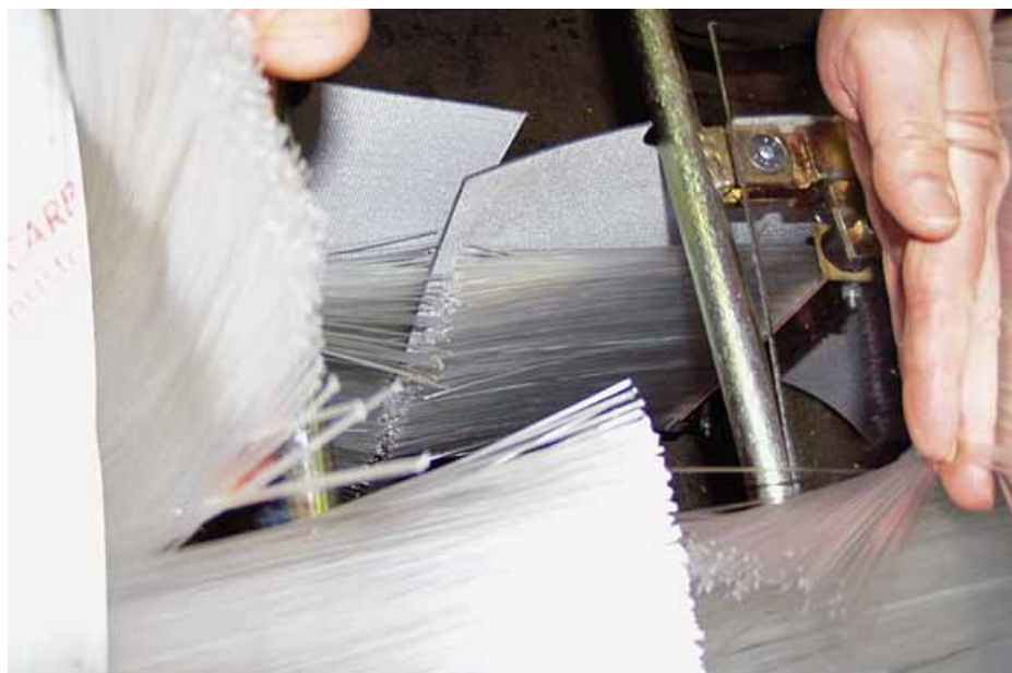
Particolare delle spazzole di umettazione brevettate dalla ditta Tecnovict, oggetto delle prove svolte presso l'azienda agricola Luigi Molinelli di Ziano Piacentino (PC). Foto Tecnovict
